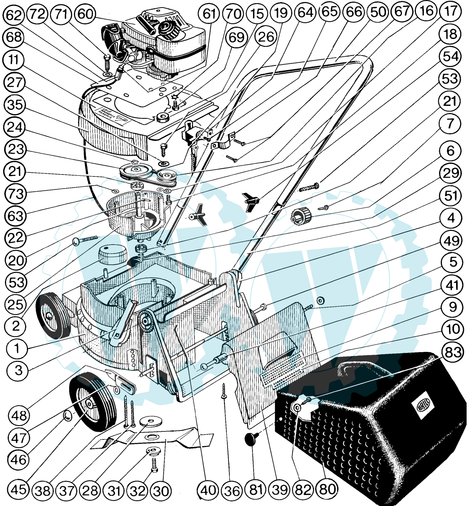
Roto - BOY H 35 TYP 1113
